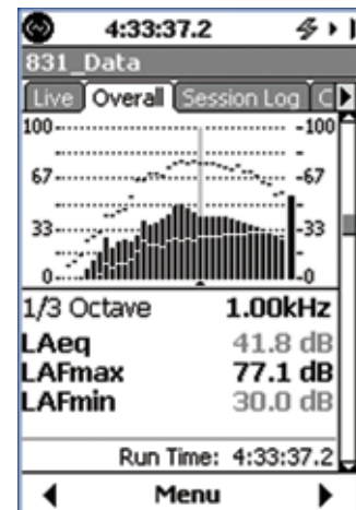
1/3 Octave Display
