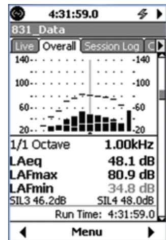
1/1 Octave Display
